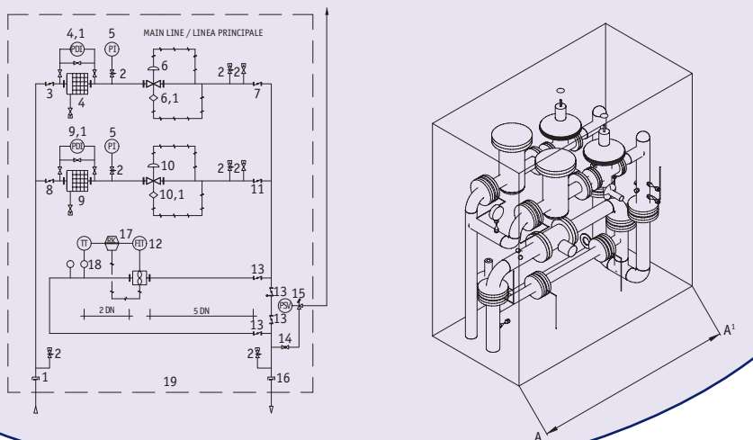
Schema di flusso e schema costruttivo P&ID and general arrangement
